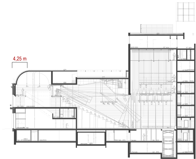
Corte longitudinal do Teatro Constantino Nery (vista Sul)
